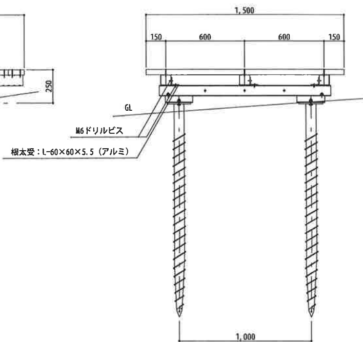
断面図 S=1:20
