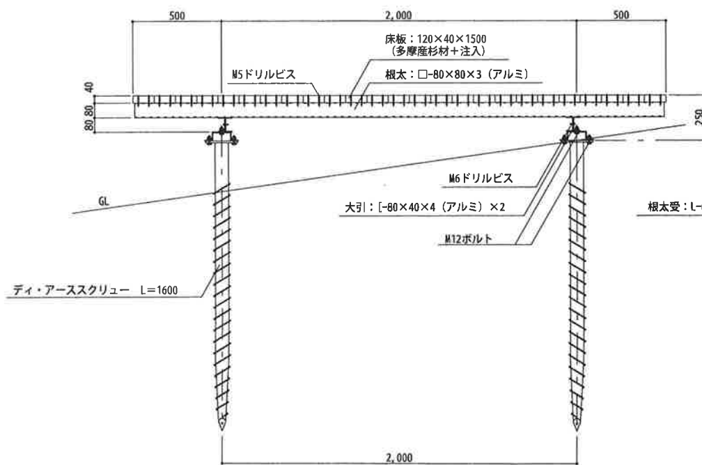
側面図 S=1:20
