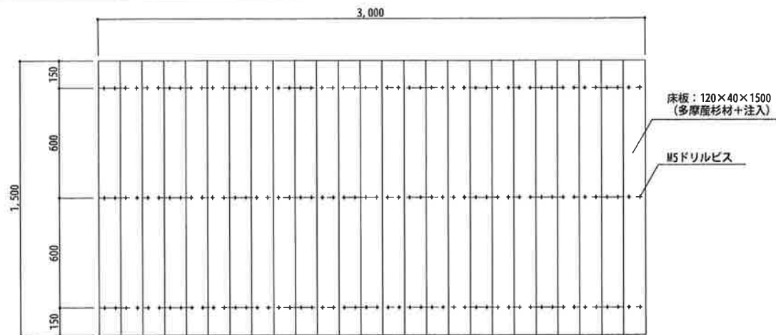
平面図 S=1:20
